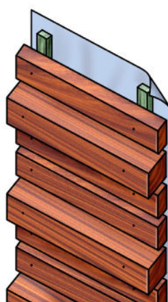
Tekening 2 Horizontale open gevelbekleding met variabele afmetingen, trapeziumvormig voor goede afwatering.
